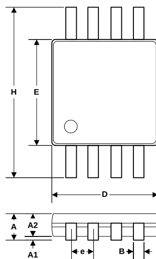
MSOP8
