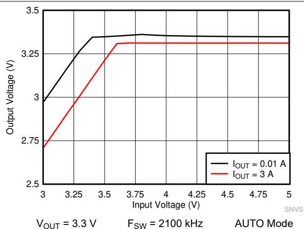
图 10-18. LM61440-Q1 Dropout Curve
