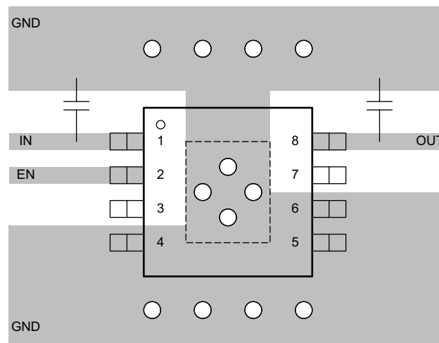
图 10-1. TPSB82-Q1 Example Layout Diagram
