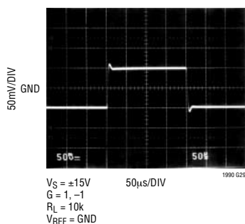
小信号瞬态响应
