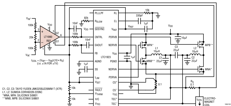
图 2：基于 PWM 的 \pm 1\text{A} 电磁电流控制器
