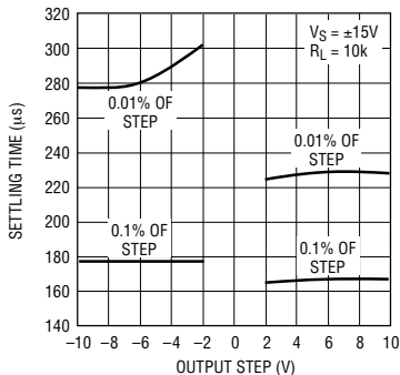
稳定时间与输出阶跃的关系曲线, G = 10
