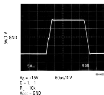
大信号瞬态响应
