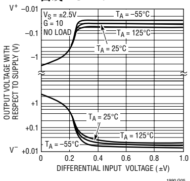
输出电压与输入电压的关系曲线, G = 10
