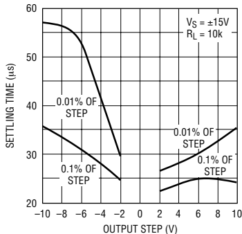
稳定时间与输出阶跃的关系曲线, G = 1
