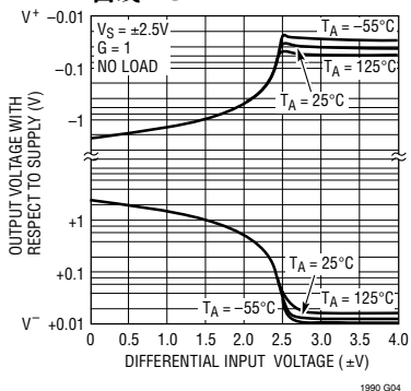
输出电压与输入电压的关系曲线, G = 1
