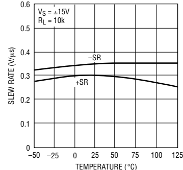
转换速率与温度的关系曲线, G = 10
