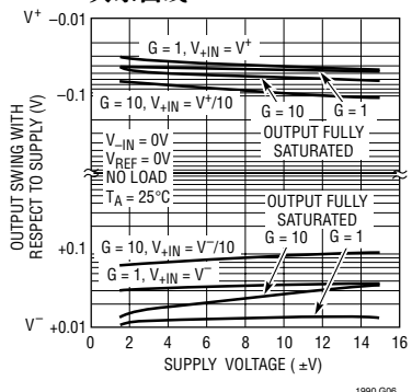
输出电压摆幅与电源电压的关系曲线
