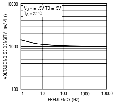
电压噪声密度与频率的关系曲线
