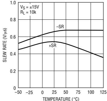
转换速率与温度的关系曲线, G = 1
