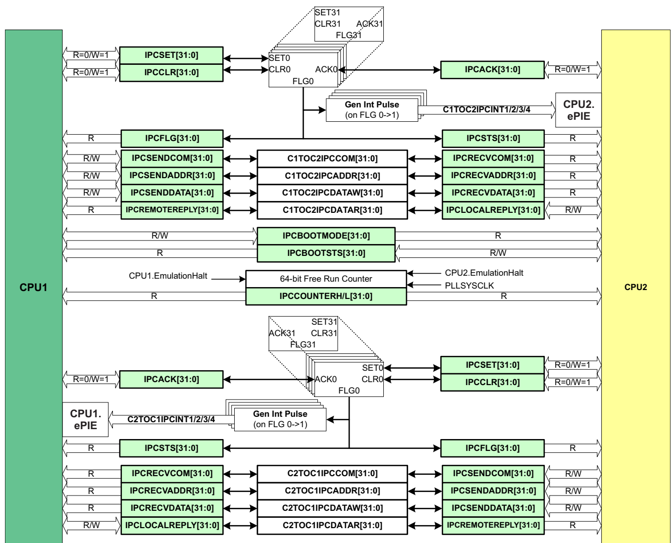
图 6-4. IPC Architecture
