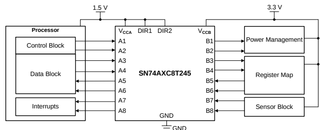
典型应用原理图
