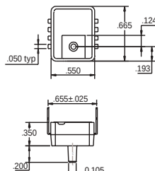
G2 Package
