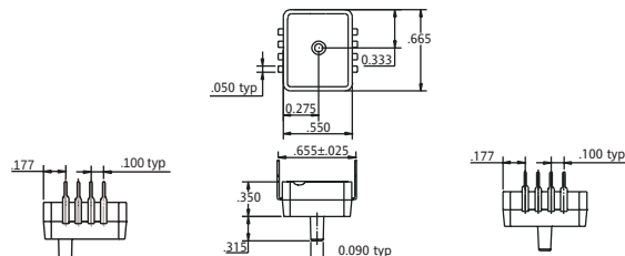
A2 Package
