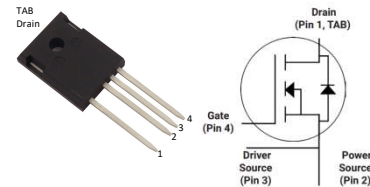
TO-247-4L
