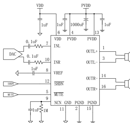
图 3-2. EG8405 典型应用图
