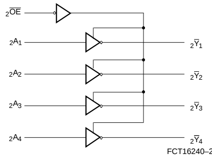
FCT16240-2
