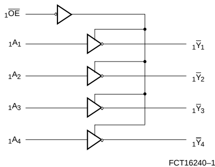
FCT16240-1
