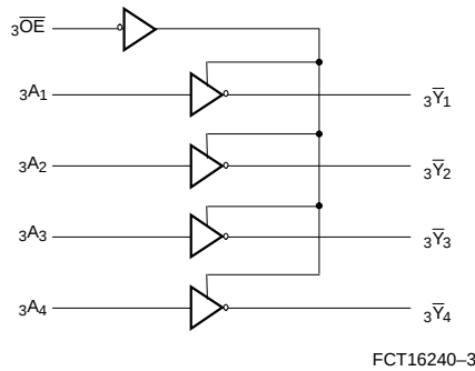
FCT16240-3
