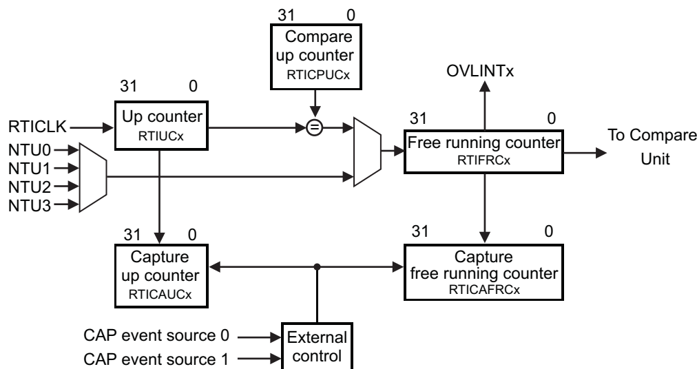
图 6-17. Counter Block Diagram
