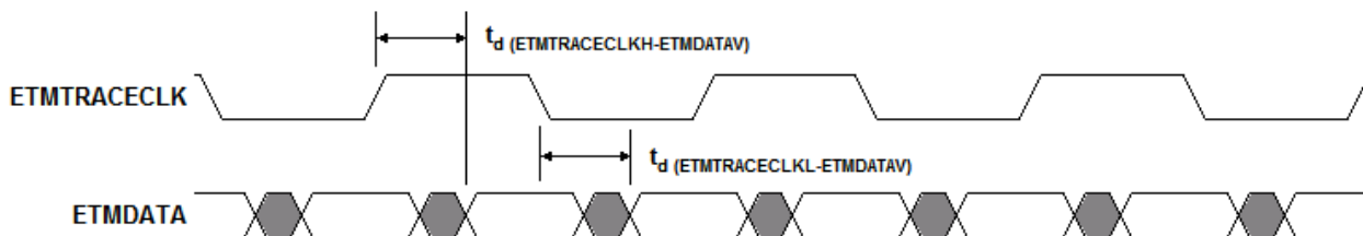
图 6-23. ETMDATA Timing
