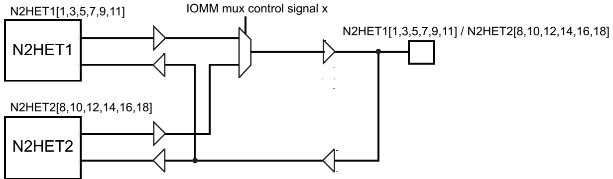
图 7-7. N2HET Monitoring
