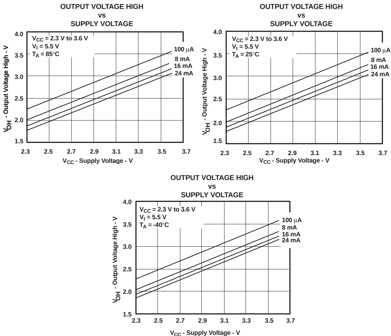
Figure 4. V_{OH} Values
