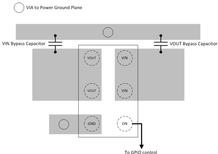
图 43. Layout Example
