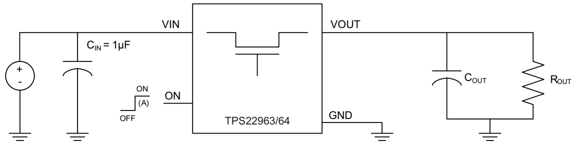
图 36. Test Circuit
