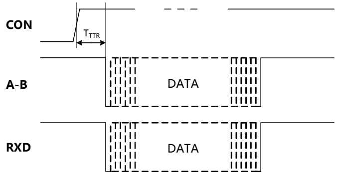
图 2. TDx01D485模块数据接收时序图
