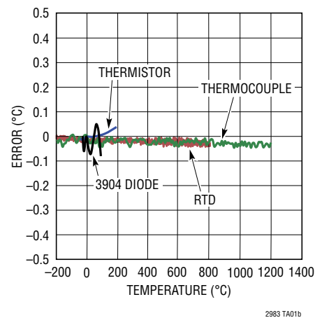
典型温度误差
