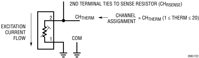
图 22：单端热敏电阻通道分配惯例
