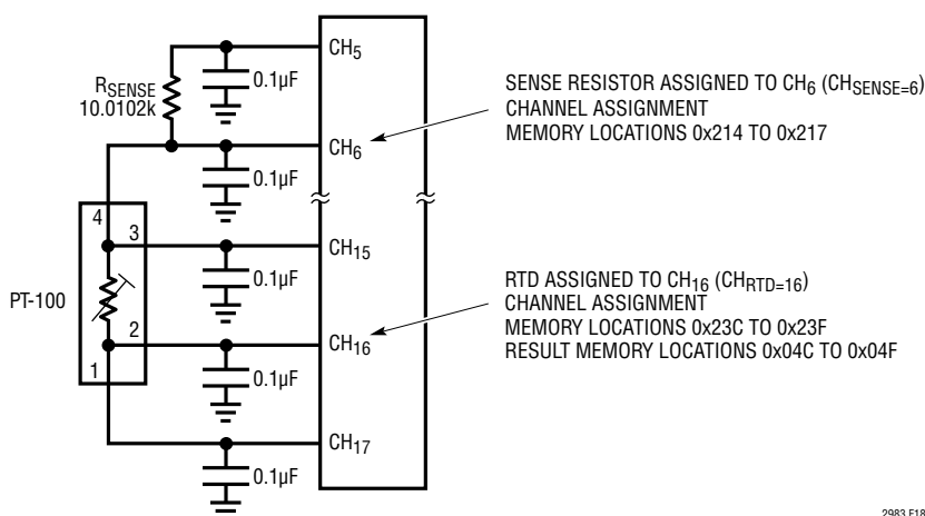
图 18：轮换型四线式 RTD 实例
