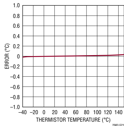
5k 热敏电阻误差与温度的关系
