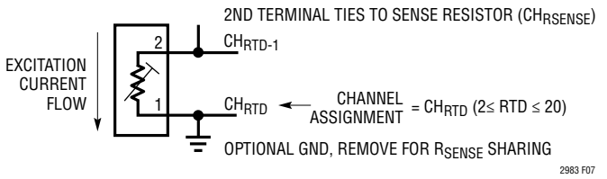
图 7：两线式 RTD 通道分配惯例
