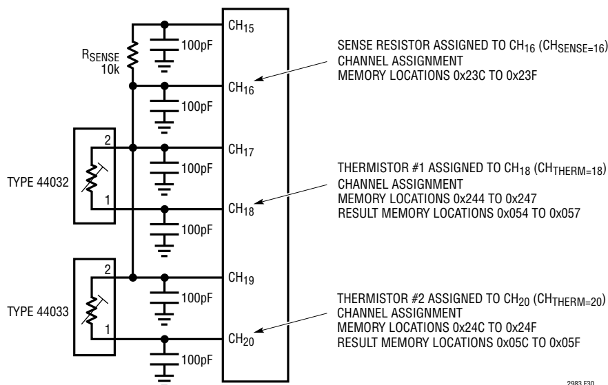
图 30：轮换和共享型热敏电阻实例
