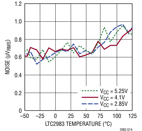
噪声与温度的关系
