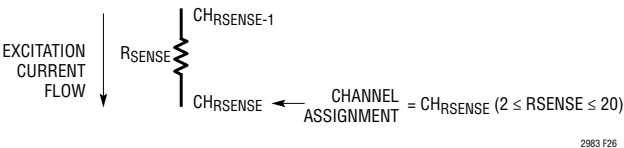
图 26：检测电阻器通道分配惯例
