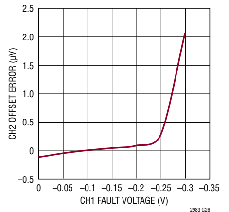
相邻通道偏移误差与输入故障电压的关系
