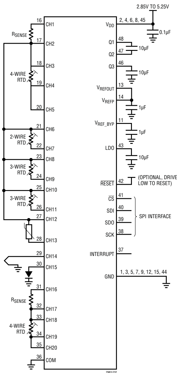
图 32：典型 RTD / 热敏电阻应用
