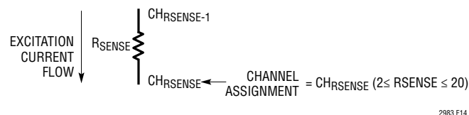
图 14：针对四线式 RTD 的检测电阻器通道分配惯例
