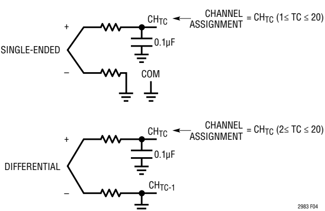
图 4：热电偶通道分配惯例
