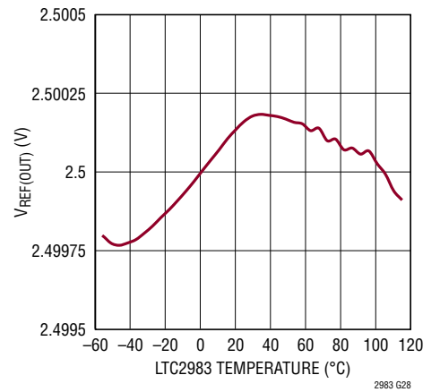
VREFOUT 与温度的关系
