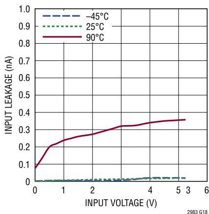
通道输入漏电流与温度的关系
