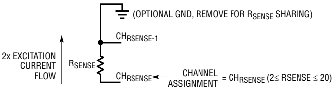
图 11：针对三线式 RTD 的三线式检测电阻器通道分配惯例
