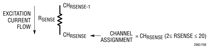
图 8：针对两线式 RTD 的检测电阻器通道分配惯例
