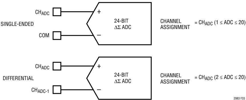
图 33：直接 ADC 通道分配惯例
