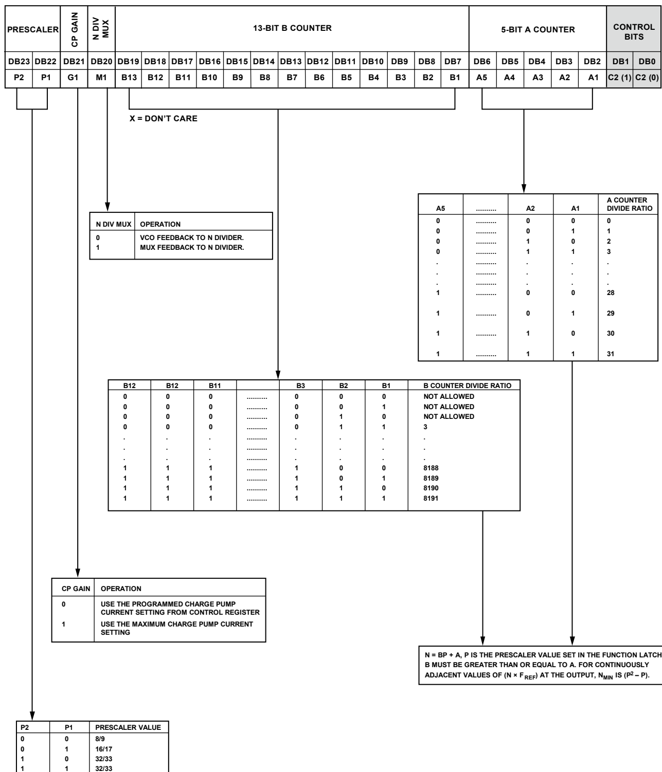
Figure 25. LO Latch
