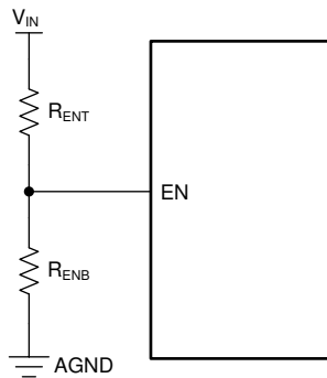
Figure 8-2. VIN UVLO Using the EN Pin
