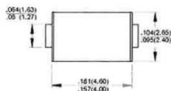
DO-214AC (SMA)
