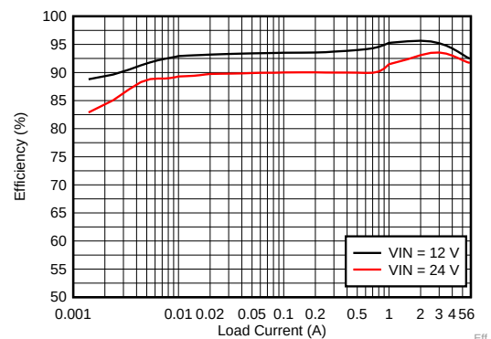
效率与负载电流 V_{OUT} = 5V , f_{SW} = 500kHz , 自动模式
