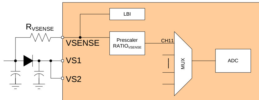
Figure 39. VSENSE Module
