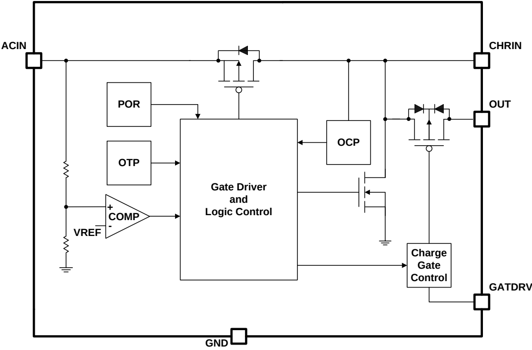
图 3 AW3210A 功能框图
