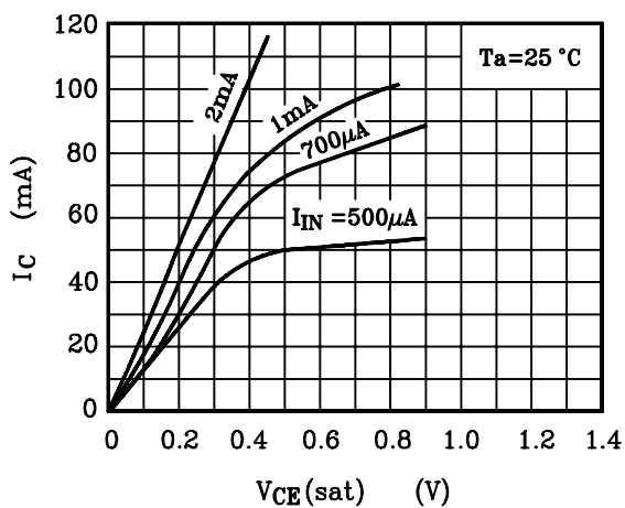
V_{CE}(\text{sat}) - I_C
