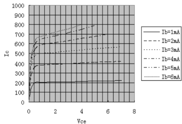
4. I_C-V_{CE}
