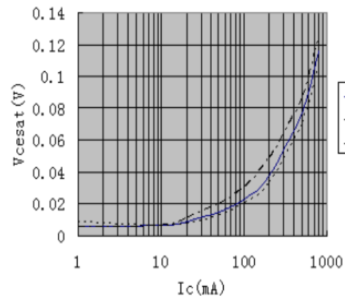
4. I_C-V_{CE}
