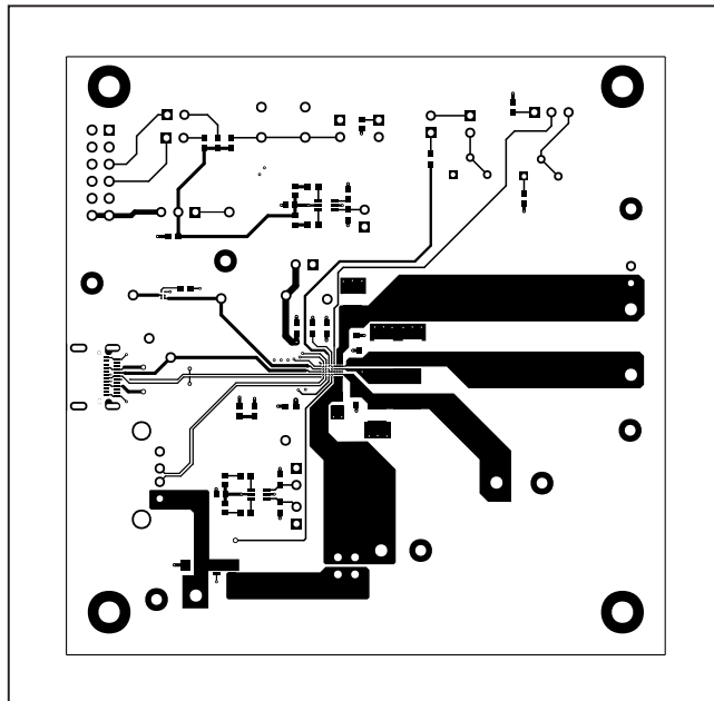
MAX14748 EV Kit—Top
