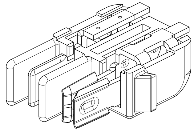
2058703-1/ 1-2058703-1 SHOWN
