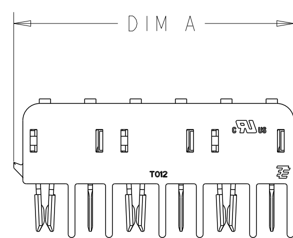
2058703-3/ 1-2078503-3 SCALE 3:1
