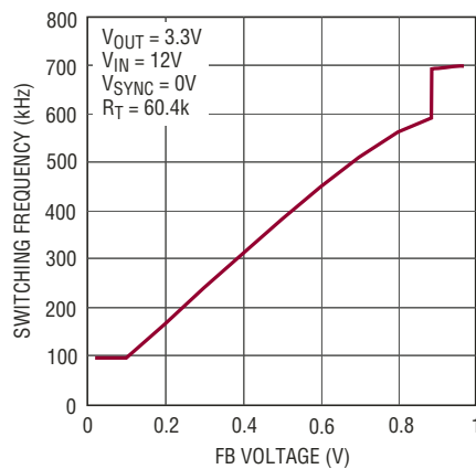
频率折返
