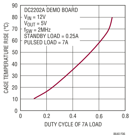
图 7：外壳温升与 7A 脉冲负载的关系曲线
