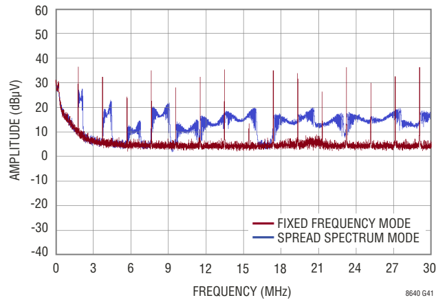
传导 EMI 性能
