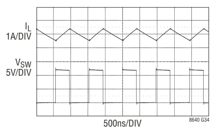
开关波形, 全频率连续操作
