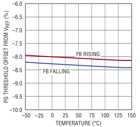
PG 低门限
