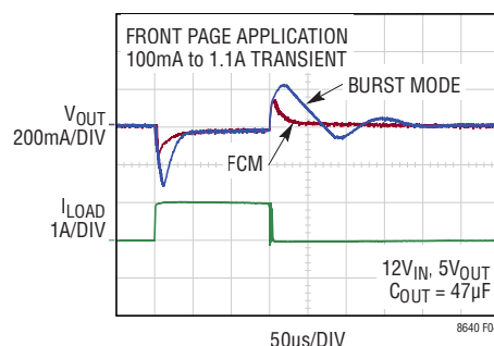
图 4：负载阶跃瞬态响应 (执行和未执行强制连续模式)
