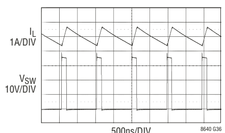
开关波形
