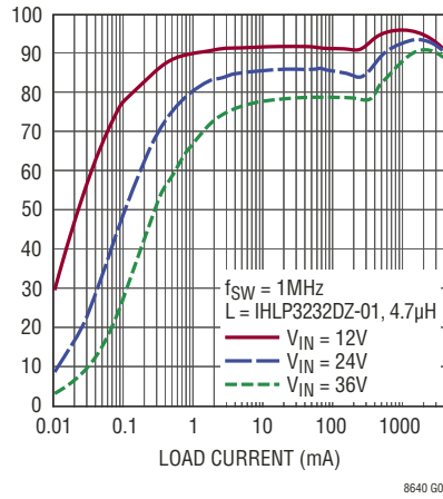
在 5V OUT 时的效率
