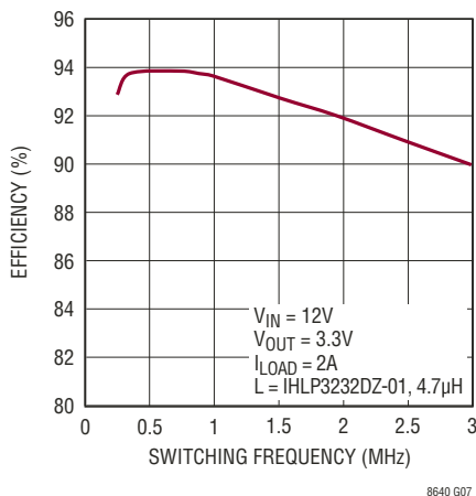
效率与频率的关系曲线
