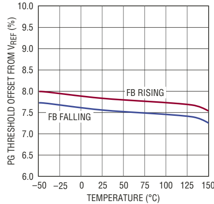
PG 高门限
