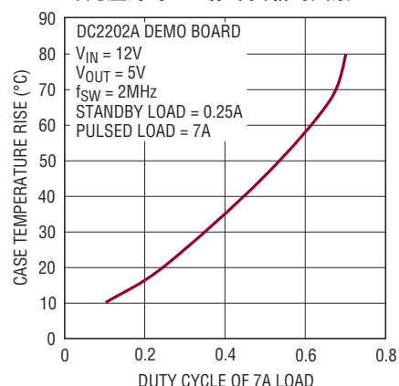
外壳温升与 7A 脉冲负载的关系
