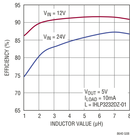
突发模式效率与电感器数值的关系
