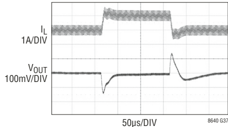
瞬态响应；负载电流 从 1A 阶跃至 2A
