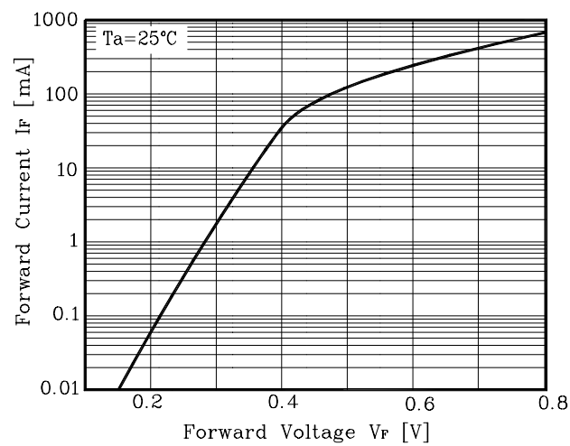
Fig. 1 I_F - V_F
