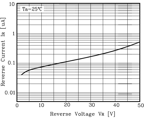
Fig. 2 I_R - V_R
