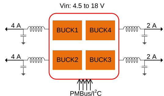
简化电路原理图
