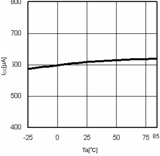
Fig.10 T_a-I_{cc}
