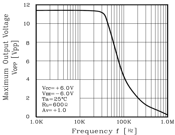
Fig. 5 V_{OP-P} vs f
