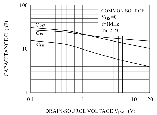
C - V_{DS}
