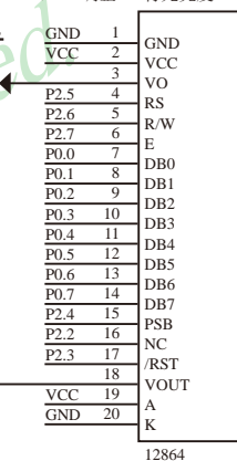
液晶模块 12864接口插座
