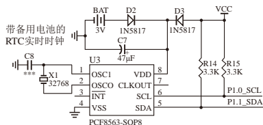
2线制I2C串行总线接口实验
