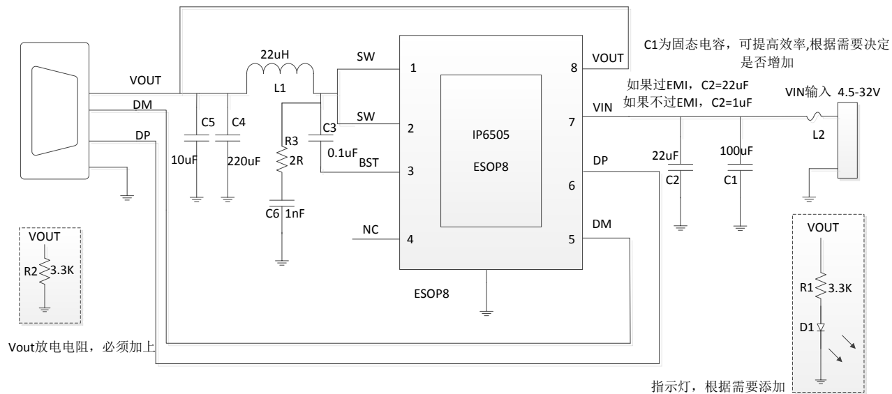
图 5 IP6505 输出应用原理图
