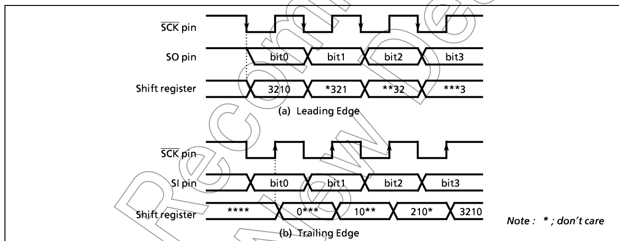
Figure 2-34. Shift Edge
