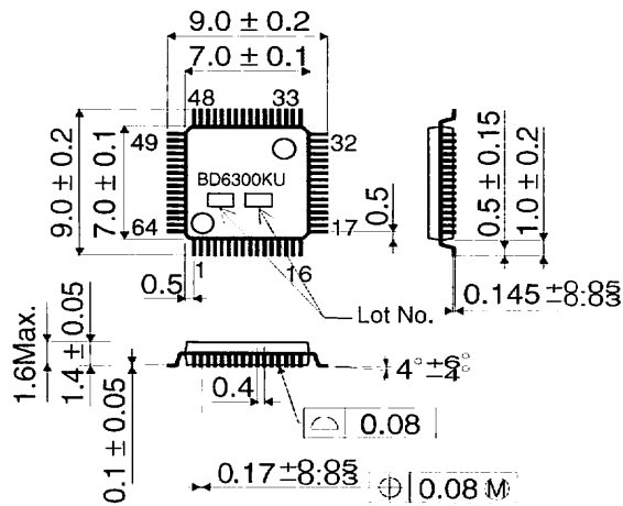
UQFP64 (Unit:mm)
