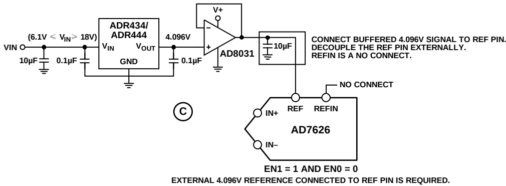
图37. 施加于REF引脚的4.096 V外部基准源
