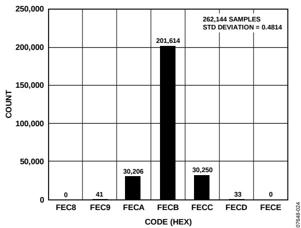
图 23. 一个直流输入的262,144次转换的直方图 (码中心、外部基准源)
