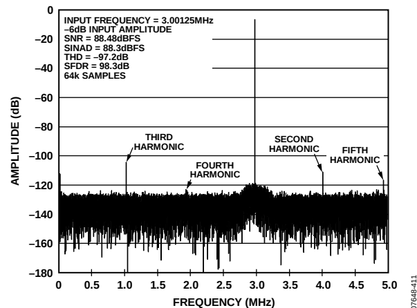
图10. FFT 3 MHz -6 dB输入音宽视图
