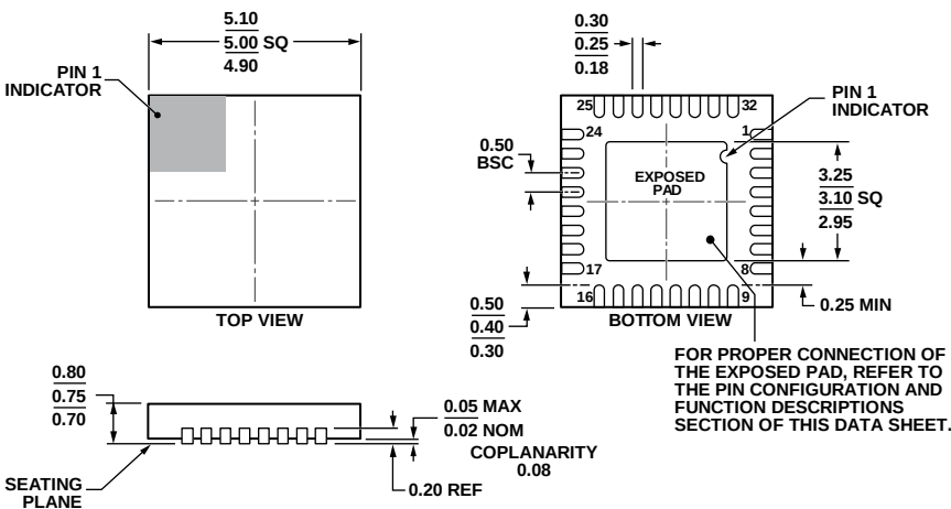
图44. 32引脚架构芯片级封装[LFCSP_WQ] 5 mm x 5 mm超薄体 (CP-32-7) 尺寸单位: mm
