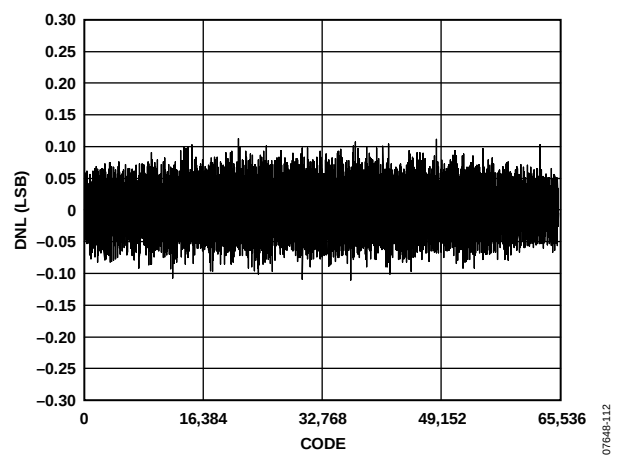
图25. 差分非线性与代码的关系(温度为25℃)
