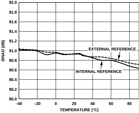
图20. SINAD与温度的关系(-0.5 dB、20 kHz输入音)
