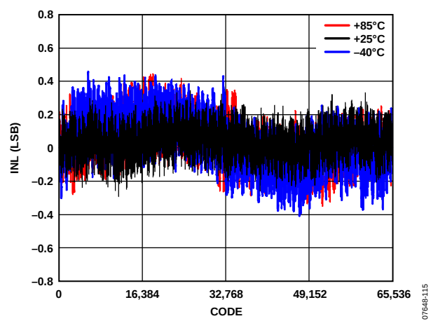
图26. 积分非线性、代码、温度三者之间的关系
