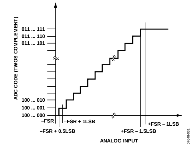
图28. AD理想传输函数(FSR表示满量程范围)
