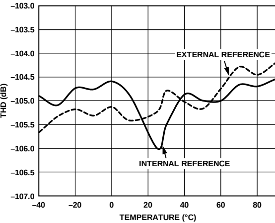
图19. THD与温度的关系(-0.5 dB、20 kHz输入音)
