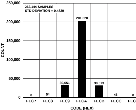
图 22. 一个直流输入的262,144次转换的直方图 (码中心、内部基准源)
