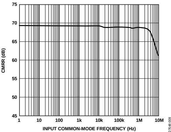
图30. 模拟输入CMRR与频率的关系
