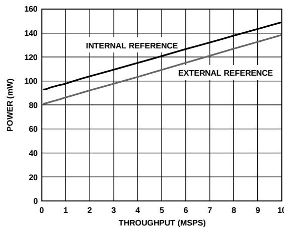
图40. 功率消耗与采样速率的关系
