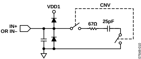
图29. 等效模拟输入电路
