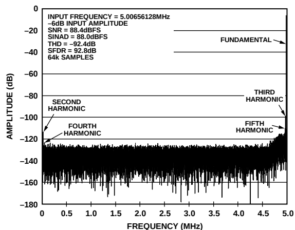
图12. FFT 5 MHz -6 dB输入音宽视图
