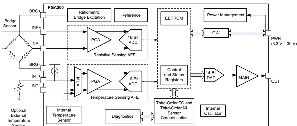
PGA300 简化框图
