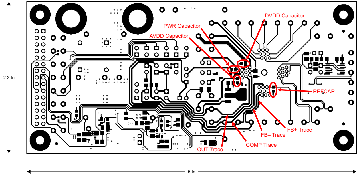
图 44. Layout Diagram
