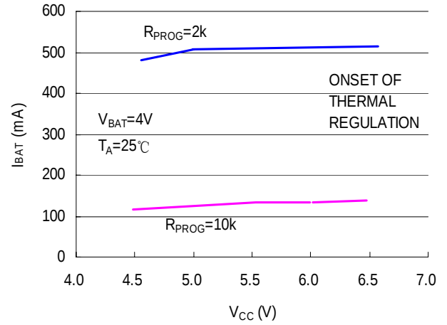
充电电流与电压关系曲线
