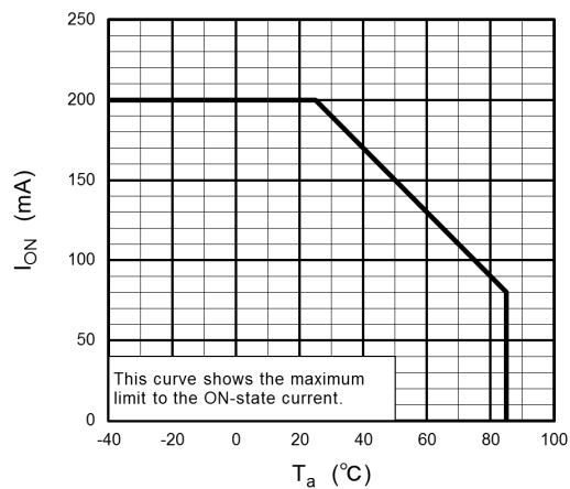
Fig. 12.1.2 I_{ON} - T_a
