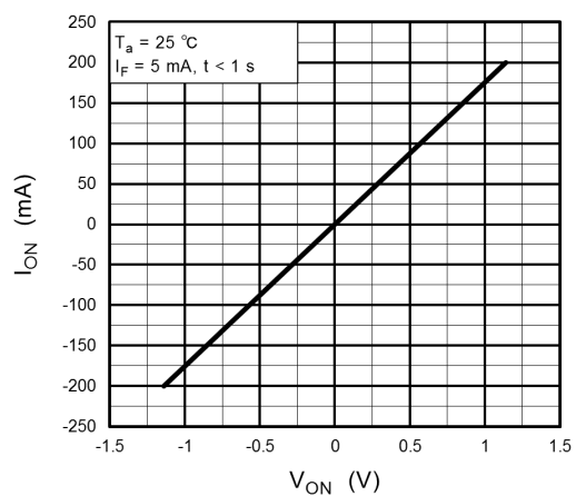
Fig. 12.1.4 I_{ON} - V_{ON}
