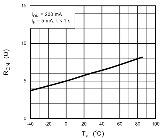
Fig. 12.1.5 R_{ON} - T_a
