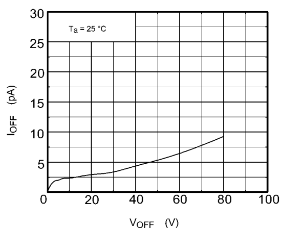
Fig. 12.1.9 I_{OFF} - V_{OFF}
