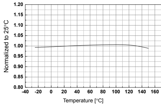
SoftStart Voltage vs. Temp.
