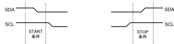
图 16-3. START 和 STOP 条件
