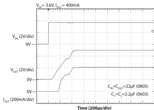
Startup (400mA)
