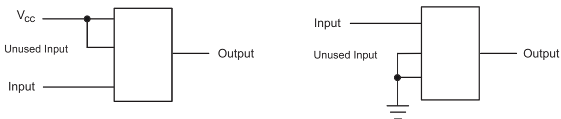
图 11-1. Layout Diagram
