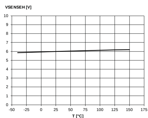
Figure 27: Vsenseh vs. Tcase
