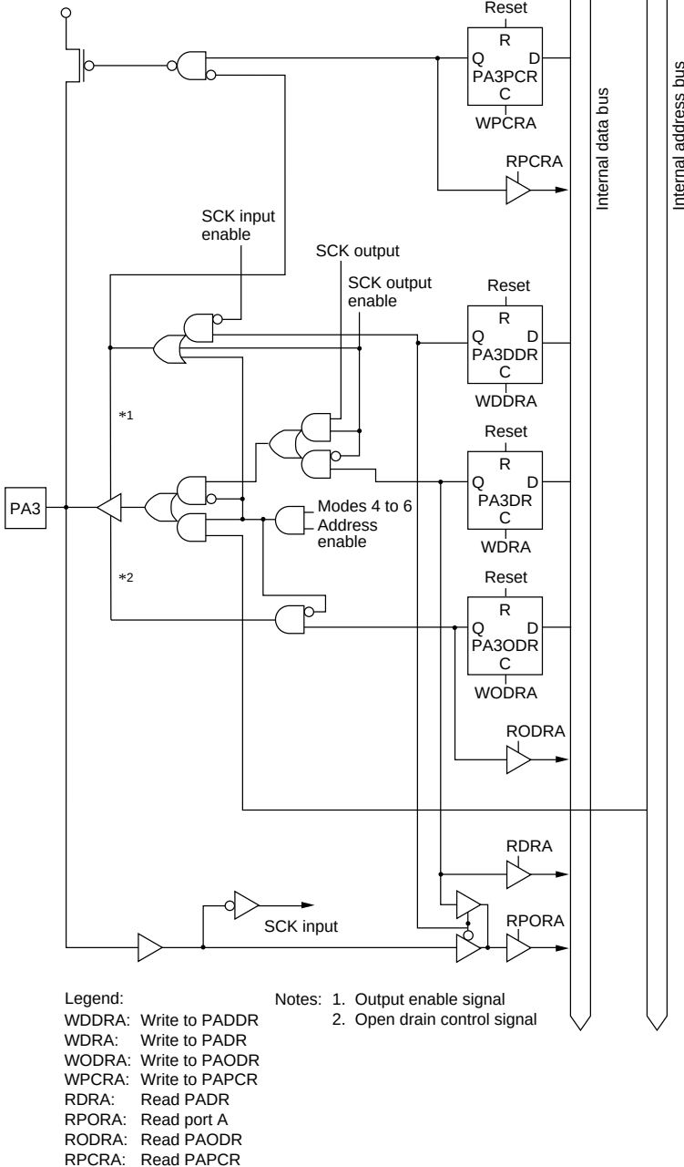
Figure C.18 (d) Port A Block Diagram (Pin PA3)
