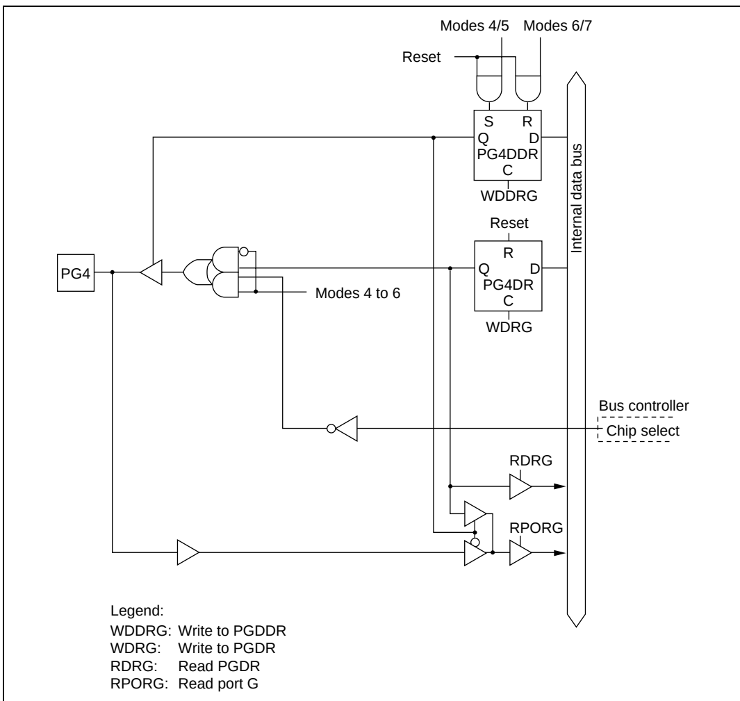
Figure C.12 (d) Port G Block Diagram (Pin PG4)
