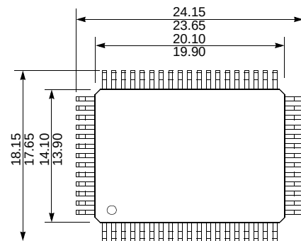
64MQFP
