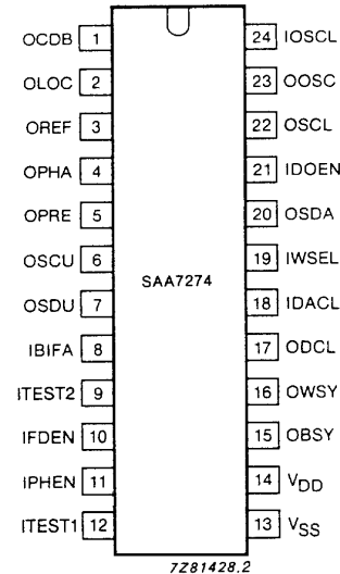
Fig.2 Pinning diagram.
