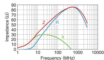
KMZ1608RHR600ATD25
