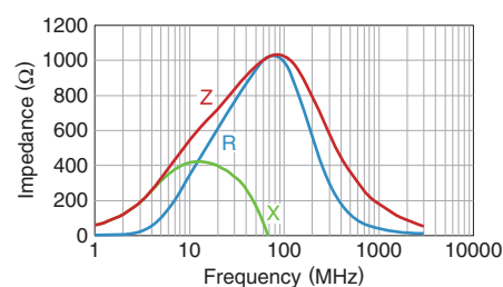
KMZ1608RHR102ATD25
