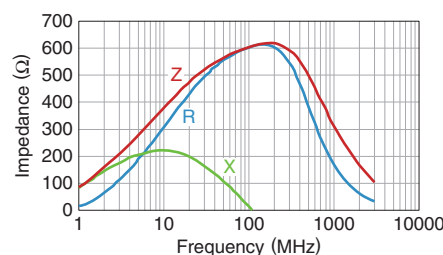
KMZ1608BHR601CTDH5
