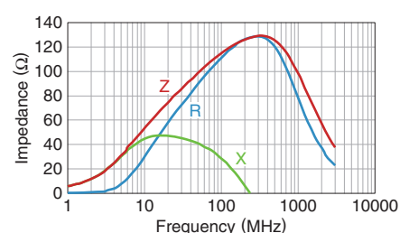
KMZ1608RHR121ATD25
