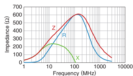
KMZ1608RHR601ATD25
