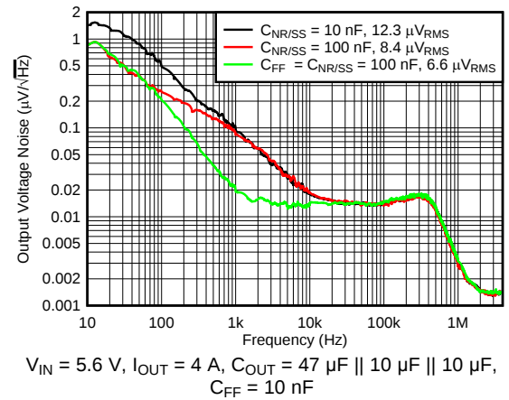
图 16. Output Noise at 5.0-V Output vs C_{NR/SS} and C_{FF}
