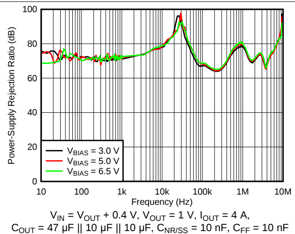
图 10. V_{BIAS} PSRR vs Frequency
