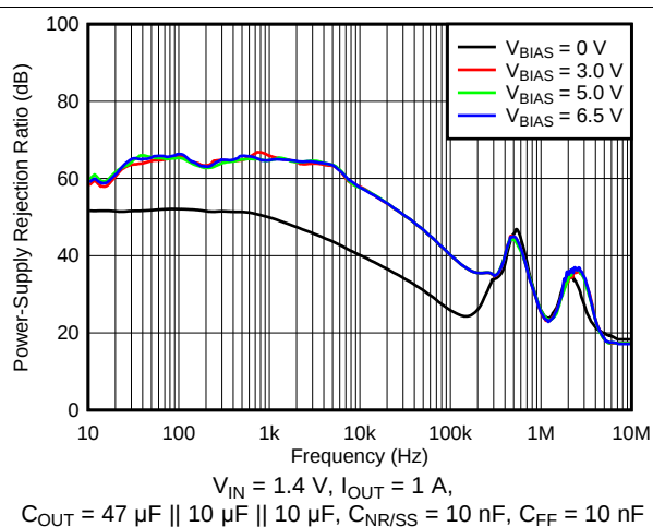
图 3. PSRR vs Frequency and V_{BIAS}
