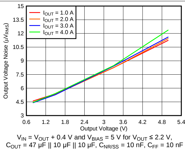
图 11. Output Voltage Noise vs Output Voltage
