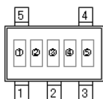
SOT-25
